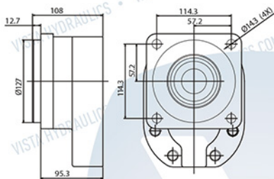
SAE C 4 furos, ø piloto 127 mm (5")
