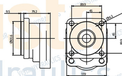
SAE B 4 Furos, ø Piloto 101.6mm(4")
