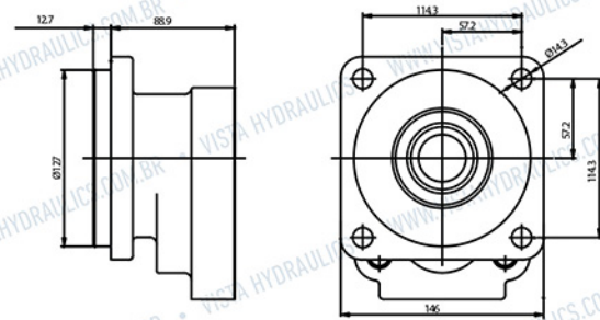
SAE B 4 Furos, ø Piloto 127mm (5")
