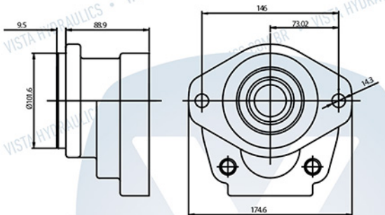
SAE B 2 Furos, \phi Piloto 101,6mm (4")
