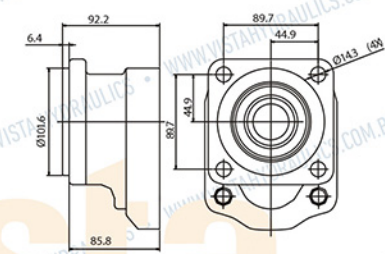
SAE B 4 furos, ø piloto 101,6 mm (4")
