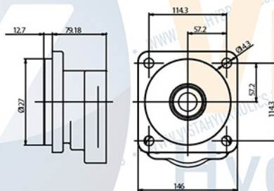
SAE B 4 Furos, ø Piloto 127mm(5")
