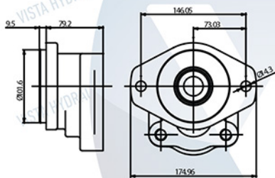
SAE B 2 Furos, ø Piloto 101.6mm(4")
