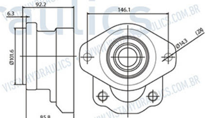
SAE B 2 furos, ø piloto 101,6 mm (4")
