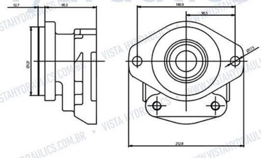
SAE C 2 Furos, \phi Piloto 127mm (5")
