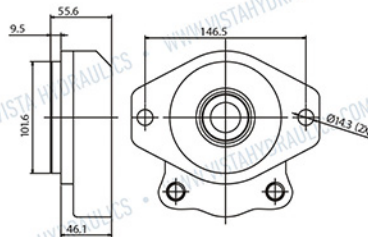
SAE B 2 furos tipo curta, ø piloto 101,6 mm (4")
