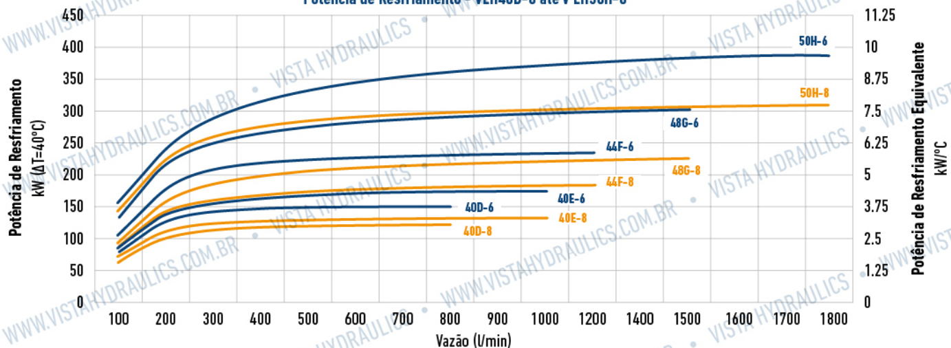
Potência de Resfriamento - VEH40D-6 até V EH50H-6
