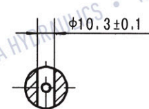
Eixo H Eixo cilíndrico Ø25.4 Com furo na ponta de Ø10.3
