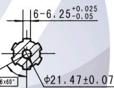
Eixo S Eixo estriado SAE 6 dentes
