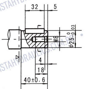
Eixo J Eixo cilíndrico Ø25 Chaveta paralela 7x7x32
