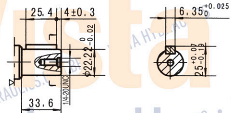
Eixo D Eixo cilíndrico Ø22.22 Chaveta paralela 6.35x6.35x25.4
