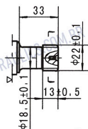
Eixo I Eixo estriado 13 dentes DP16/32
