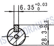
Eixo K Eixo cilíndrico Ø25.4 Chaveta woodruff (meia lua) Ø25.4x6.35
