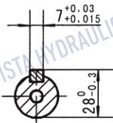
Eixo J Eixo cilíndrico Ø25 Chaveta paralela 7x7x32
