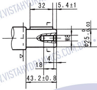
Eixo A Eixo cilíndrico Ø25 Chaveta paralela 8x7x32
