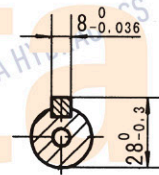
Eixo P Eixo cilíndrico Ø25 Chaveta paralela 8x7x25
