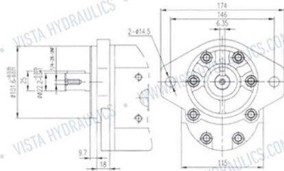
P16 (Eixo 7/8" chavetado)
