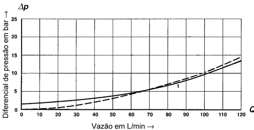
Curvas \Delta p -Q
