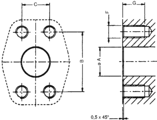
Flange SAE (3000 PSI)
